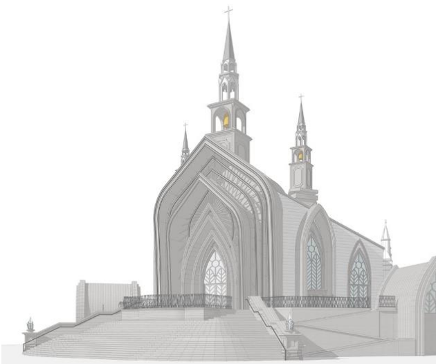
ภาพที่ 6 ทศนิยมภาพด้านหน้าภายนอกโบสถ์ ด้วยโปรแกรม Sketch up และ โปรแกรม 3Ds Max ที่มา : เอกพงษ์ ตรีตรง
