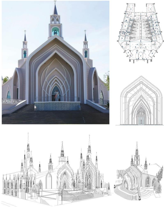
ภาพที่ 9 ทศนียภาพภายนอกโบสถ์ และรูปด้านภายในโบสถ์ด้วยโปรแกรม Sketch up และ โปรแกรม 3Ds Max ที่มา : เอกพงษ์ ตรีตรง
