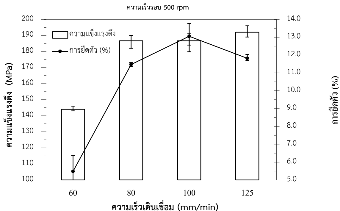
ภาพที่ 9 ความสัมพันธ์ความแข็งแรงดึงความเร็วรอบ 500 รอบต่อนาที
