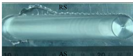
(ข) ผิวหน้ารอยเชื่อมความเร็วรอบ 500 รอบต่อนาที ความเร็วเดินแนวเชื่อม 125 มม./นาที
