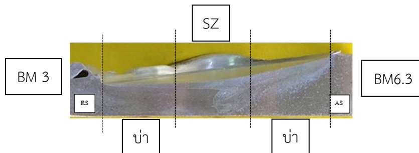
ภาพที่ 12 การผสมกันรวมที่ความเร็วรอบ 500 รอบต่อนาที ความเร็วเดินแนวเชื่อม 125 มม./นาทึ
