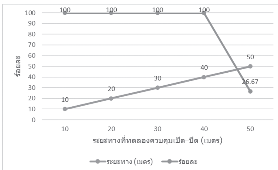
รูปที่ 7 กราฟแสดงค่าร้อยละการทดสอบควบคุม เปิด - ปิด ในระยะทางที่ต่างกัน
